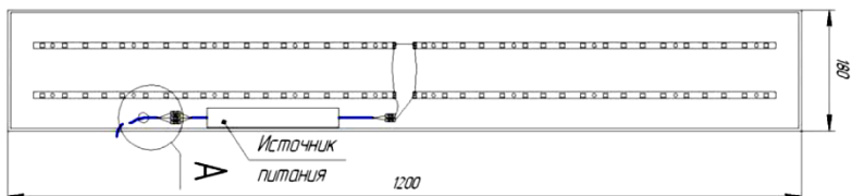
Рис.1 Светильник Офис Люкс 2x36
