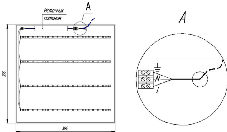
Рис.2 Светильник Офис Люкс 4x18
